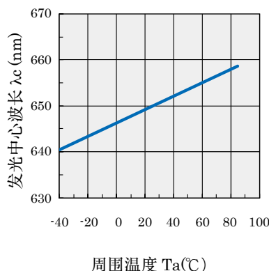
图 8. 发光中心波长温度特性
