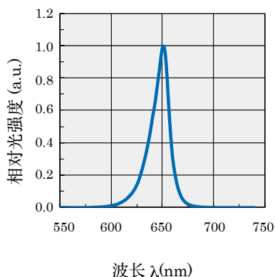
图 7. 发光光谱
