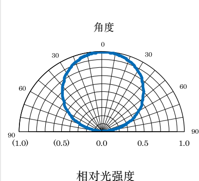
图 6. 指向特性
